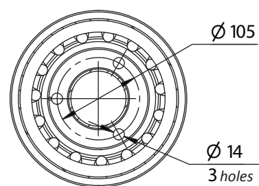
A-A (1:5)
